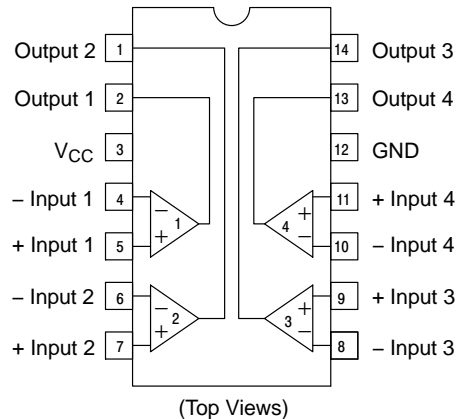
SOIC-14 / TSSOP-14
